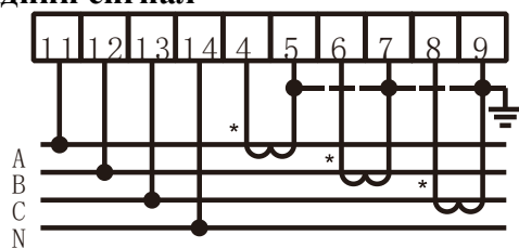
3-фазний 4-провідний вхід (3P4W)
