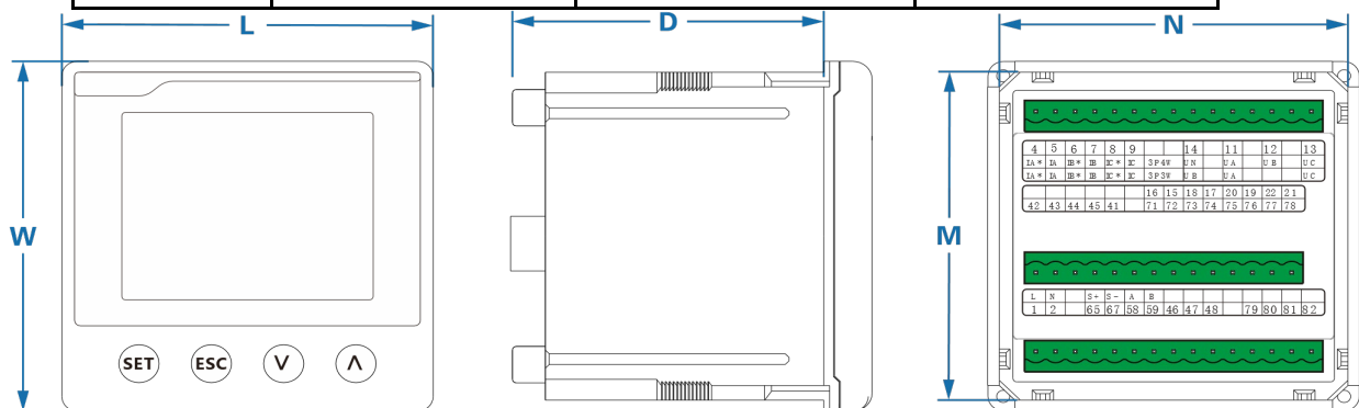
Рисунок 8 Розмірна схема
