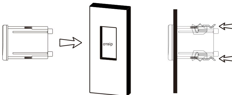
Рисунок 9 Схема встановлення
