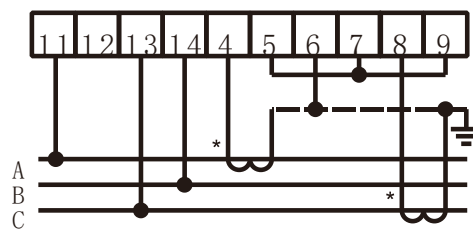
3-фазний 3-провідний вхід (3P3W)
